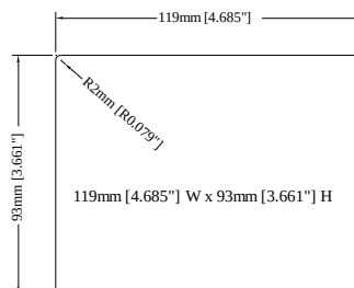
Cutout Dimensions
